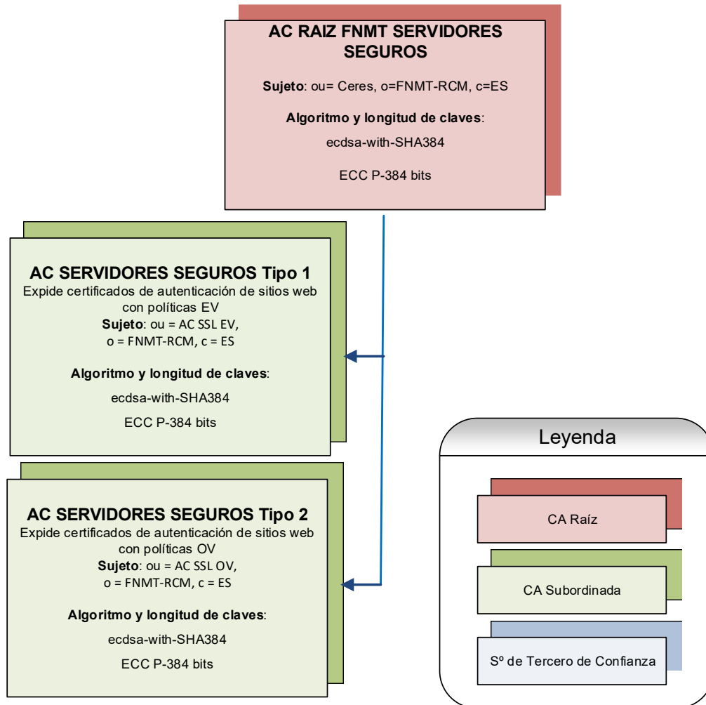
Figura-2: Jerarquía de AC RAIZ FNMT-RCM SERVIDORES SEGUROS
