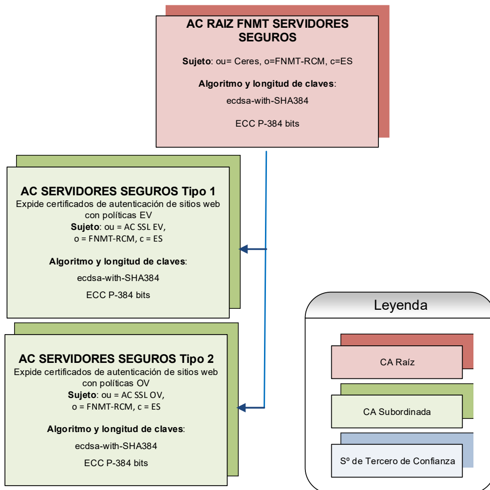
Figura-1: Jerarquía de AC RAIZ FNMT-RCM SERVIDORES SEGUROS
